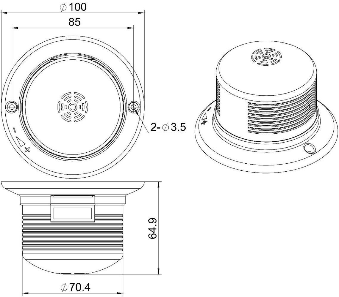
LK210 报警器尺寸图:
