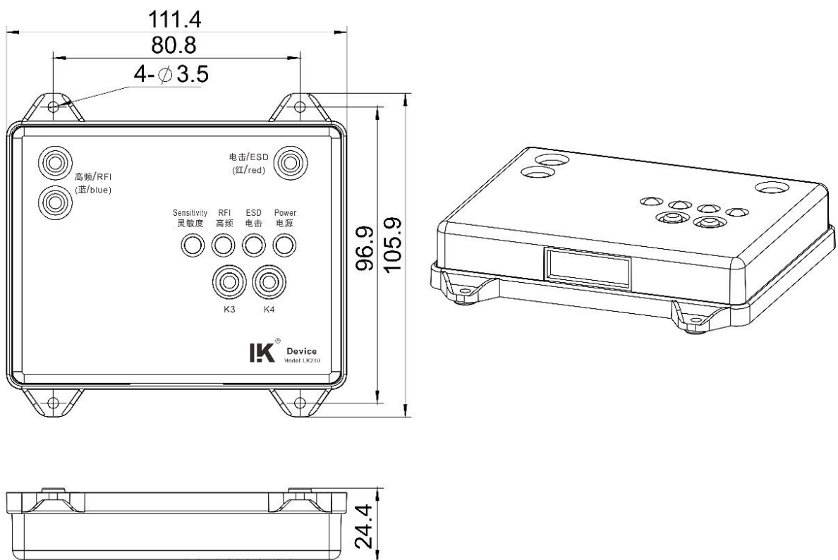
LK210 分机尺寸图:
