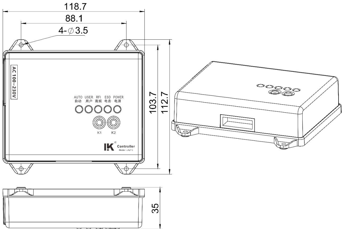
LK210 主机尺寸图:
